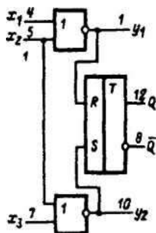
Условное графическое обозначение К114ТР1
