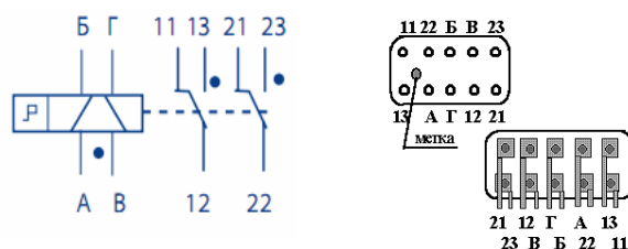
Схема электрическая принципиальная РПС 45, РПС 45-1
