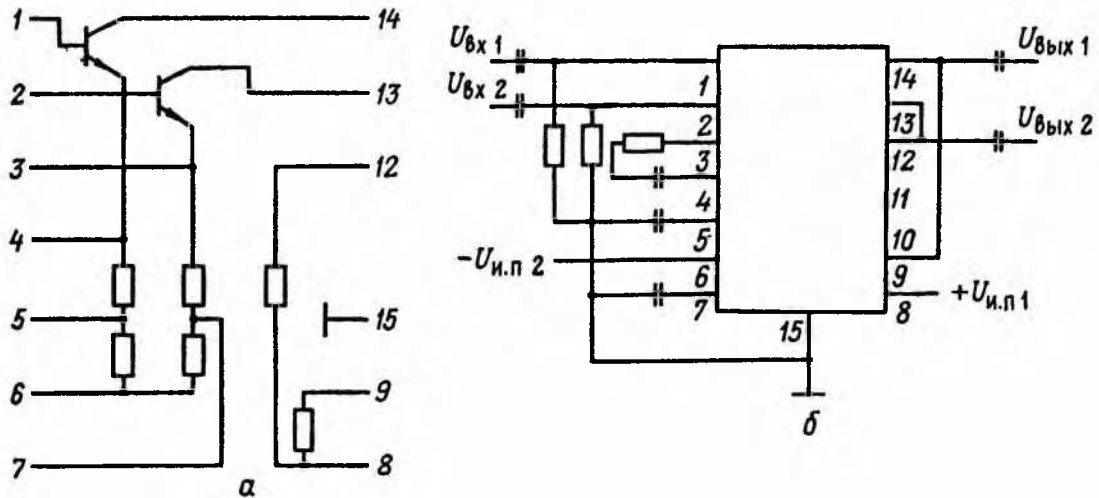
Принципиальная схема ИМС 228УВ4, К228УВ4 (а) и пример ее использования в балансном усилителе (б)
