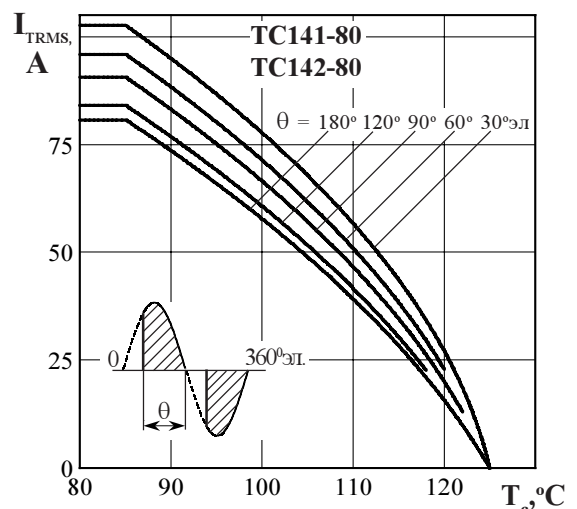
Рисунок 2 - Зависимость допустимого действующего тока в открытом состоянии I_{TRMS} от температуры корпуса T_c для токов синусоидальной формы частоты f = 50\text{ Гц}
