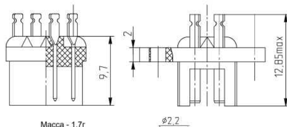
Рисунок 11 Вилка РШ2Н-1-19
