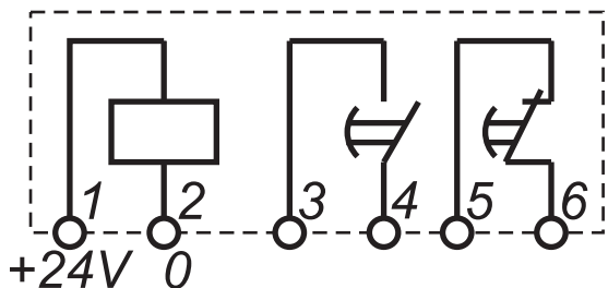
Рисунок 7 - Схема подключения ВЛ-67 на напряжение 24 В
