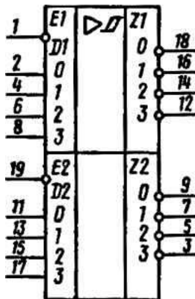
Условное графическое обозначение К555АПЗ
