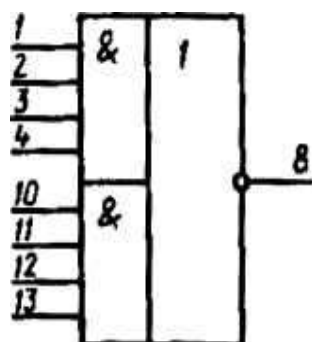
Условное графическое обозначение К555ЛР4
