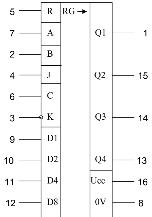
Рис. 1. Условное графическое обозначение микросхем 1526ИР9 ЭП
