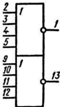
Условное графическое обозначение КР1561ЛЕ6, КФ1561ЛЕ6
