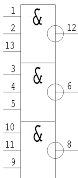
Рис. 1. Условное графическое обозначение микросхем 1564ЛА4 корпусе 401.14-5.
