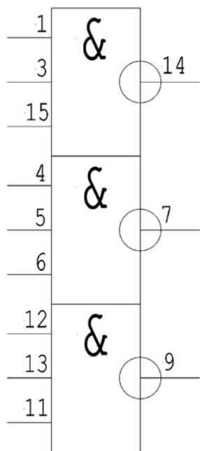
Рис. 2. Условное графическое обозначение микросхем 1564ЛА4 ЭП корпусе 5119.16-А.
