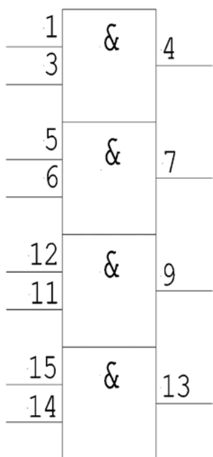
Рис. 2. Условное графическое обозначение микросхем 1564ЛИ1 ЭП в корпусе 5119.16-А.
