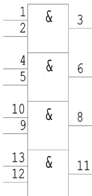
Рис. 1. Условное графическое обозначение микросхем 1564ЛИ1 ЭП в корпусе 401.14-5.
