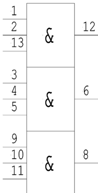
Рис. 1. Условное графическое обозначение микросхем 1564ЛИЗ ЭП в корпусе 401.14-5.
