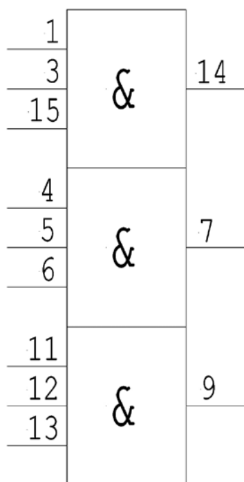
Рис. 2. Условное графическое обозначение микросхем 1564ЛИЗ ЭП в корпусе 5119.16-А.
