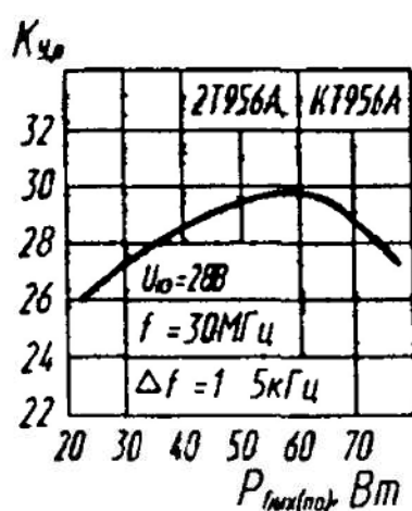
Зависимость коэффициента усиления от выходной мощности
