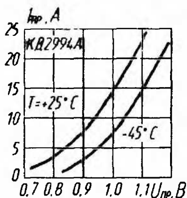
Зависимости прямого тока от напряжения
