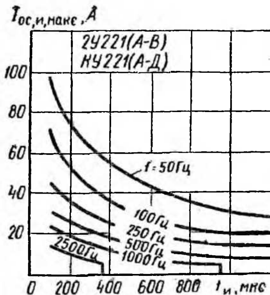
Зависимости допустимого импульсного тока в открытом состоянии от длительности импульса
