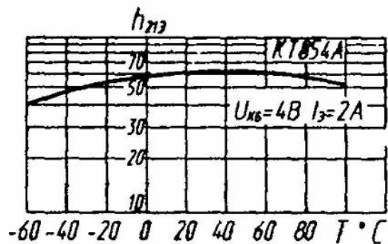
Зависимость статического коэффициента передачи тока от температуры
