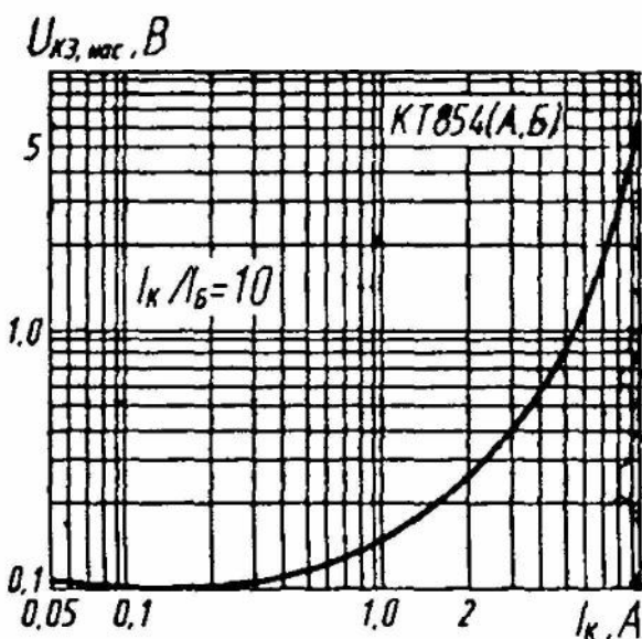
Зависимость напряжения насыщения коллектор—эмиттер от тока коллектора
