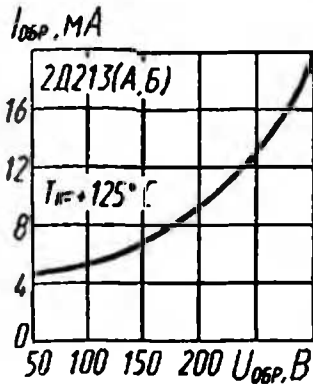
Зависимость обратного тока от напряжения
