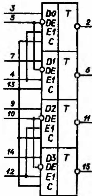
Условное графическое обозначение К500ТМ133
