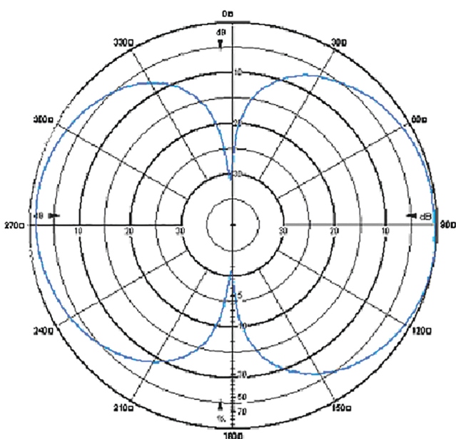
Диаграмма поляризации по горизонтали
