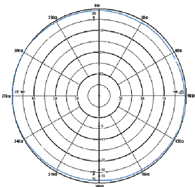
Диаграмма поляризации по вертикали
