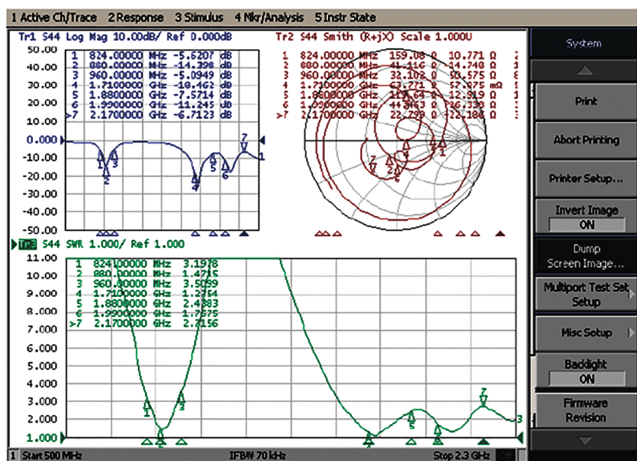
Снимок экрана АЧХ анализатора
