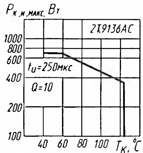
Зависимость максимально допустимой импульсной рассеиваемой мощности коллектора от температуры корпуса
