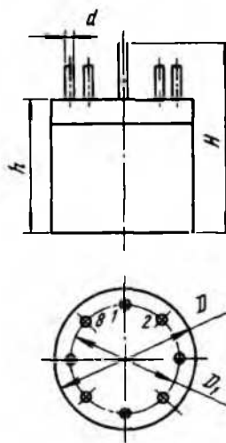
Конструктивные размеры импульсных миниатюрных трансформаторов типа ТИМ
