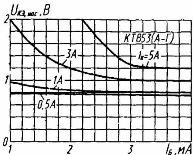
Зависимости напряжения насыщения коллектор—эмиттер от тока базы
