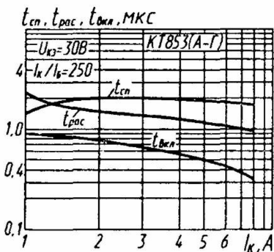
Зависимости времени спада, рассывания и включения от тока коллектора
